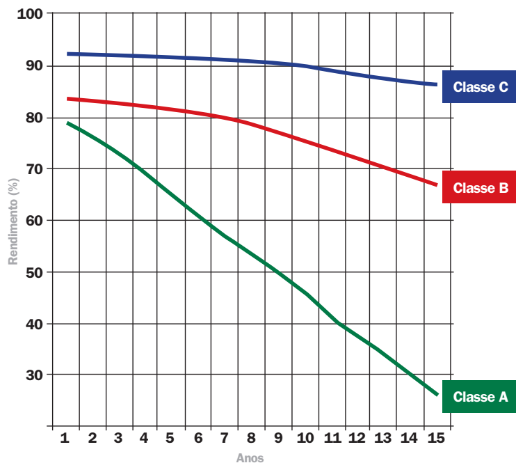
Figura 9 - Eficiência da medição em função do tempo (Nielsen et al., 2003)
