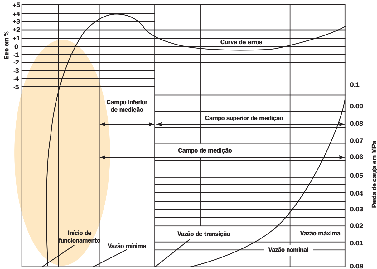
Figura 3 – Curva de Erros e Curva de Perda de Carga para hidrômetros taquimétricos para água fria
