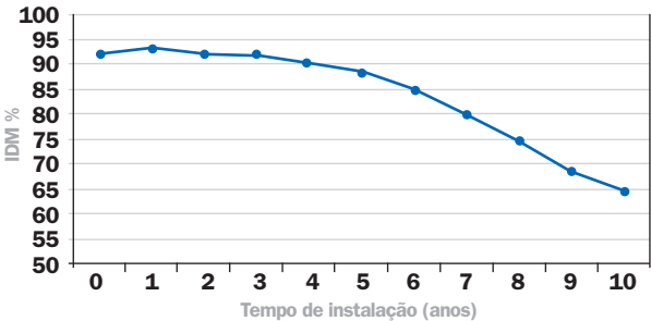
EFICIÊNCIA DA MEDIÇÃO EM FUNÇÃO DO TEMPO DE INSTALAÇÃO
