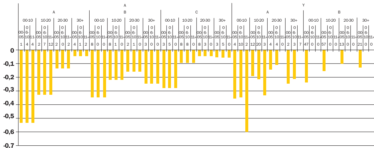
Figura 15 – Submedição por tipo de hidrômetro, classe metrológica, faixa de consumo e idade em estudo do IPT (2005). A escala de erros está em fatores unitários.
