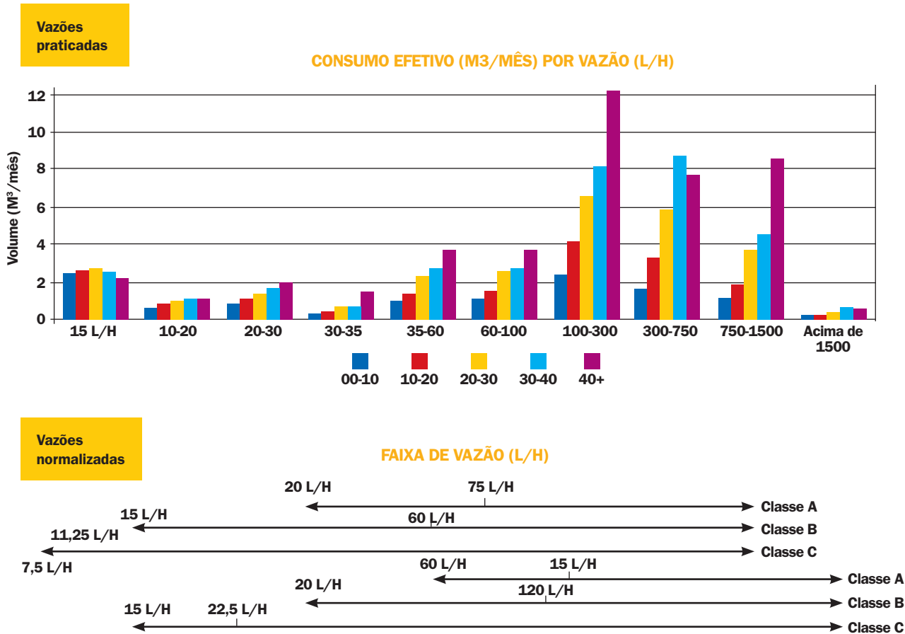
Figura 14 - Não adequação das características dos hidrômetros do mercado às vazões efetivas em consumidores do rol comum (fonte: IPT, 2005)
